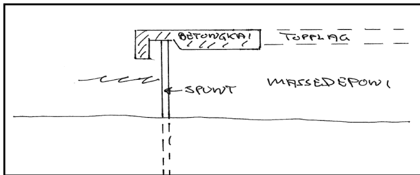
Prinssipskisse som viser oppbygging av spunt
